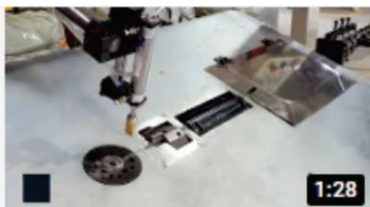
Maquina de Dobrar Arame 2D-Modelo WB-2D 408
